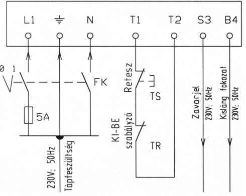
kétfokozatú égők
