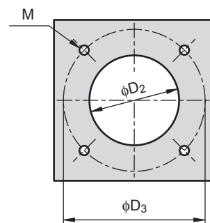
Kazánperem furatozás
