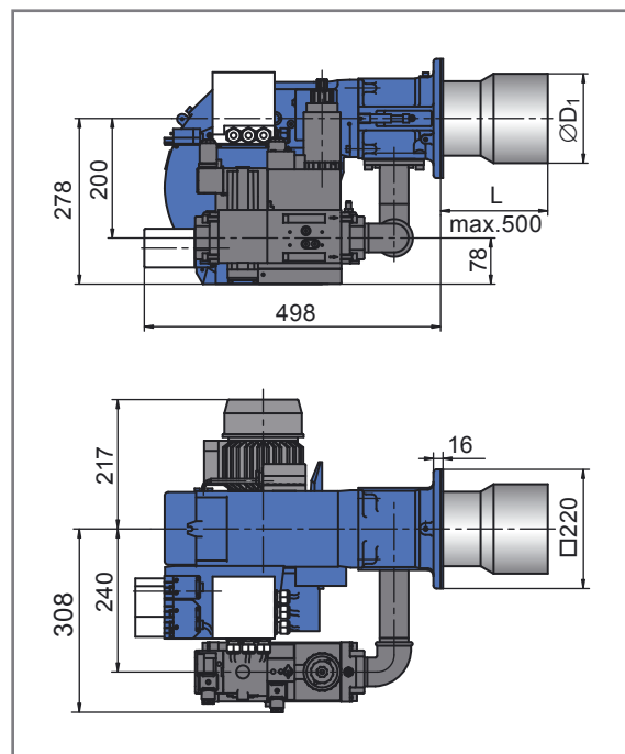
ABG-40K, ABG-45K
